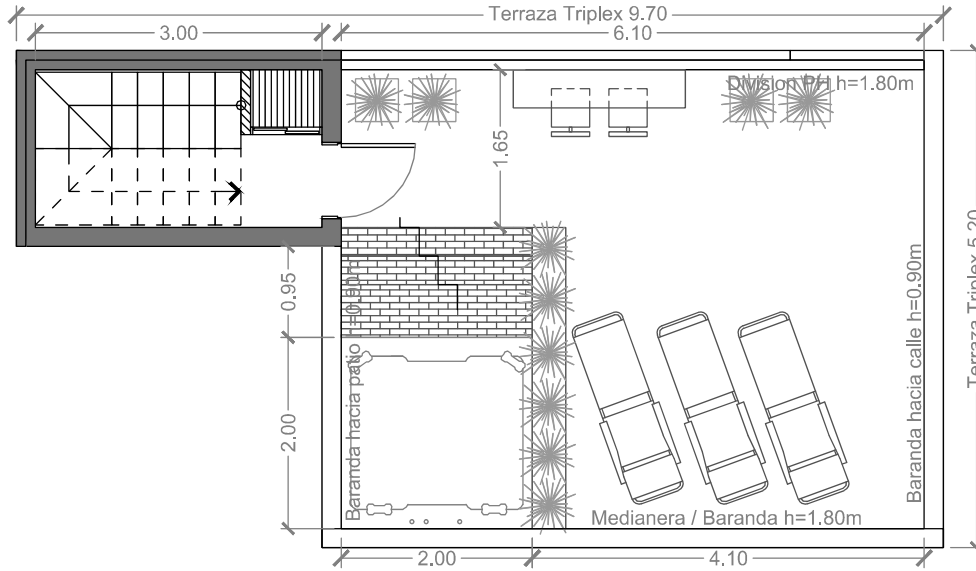
PLANTA TERRAZA
