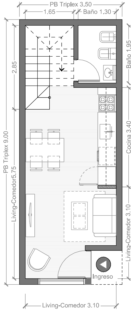
PLANTA BAJA
